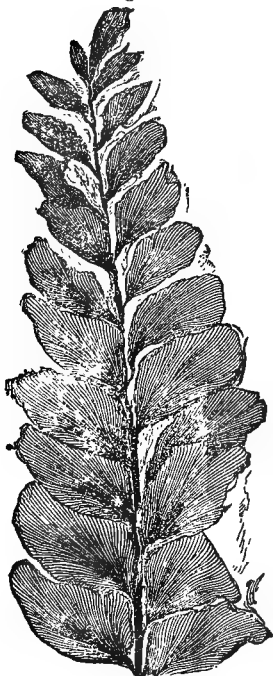
CYCLOPTERIS HIBERNICUS. (Nat. size.)
